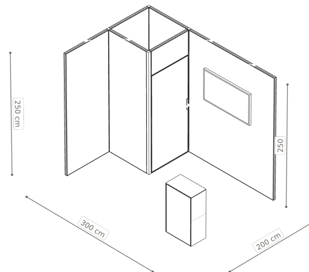
Izometria — wysokości elementów
