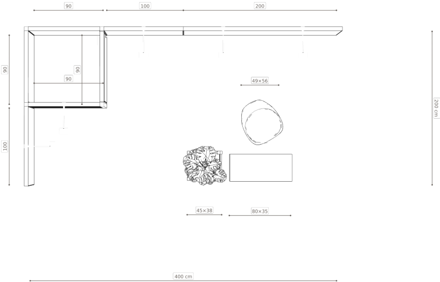
Rzut — szerokości modułów i mebli
