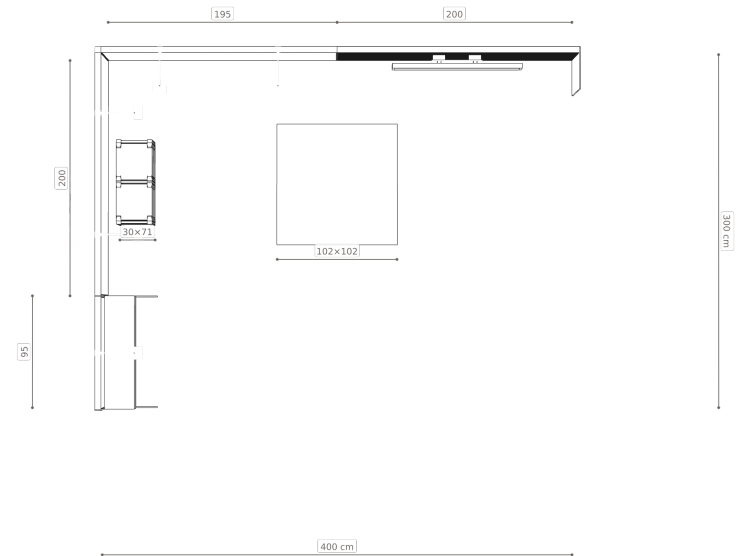
Rzut — szerokości modułów i mebli
