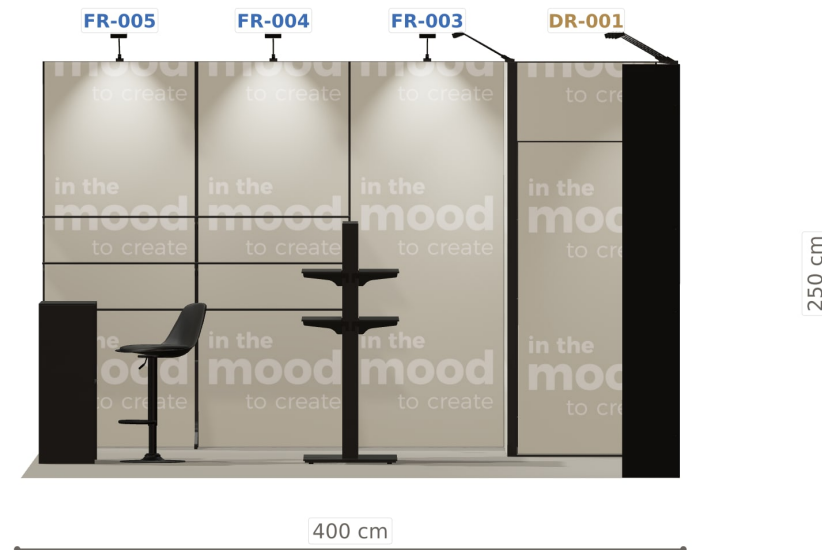
Elewacja ściany lewej
