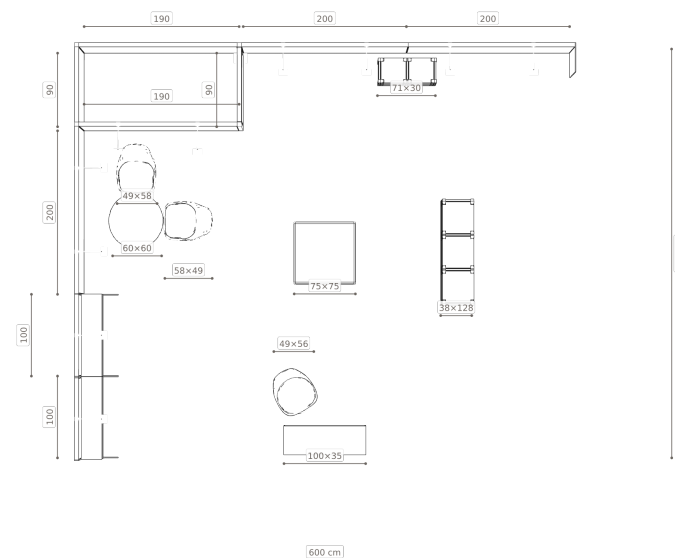
Rzut — szerokości modułów i mebli
