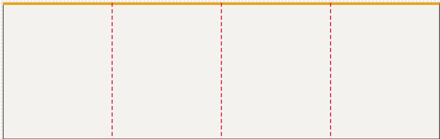
Ściana tylna od lewej: FR-002 ... FR-005, LED 801 × 250 cm plik 804 × 253 cm, spąd 1,5 cm po obrysie, łączeń: 3
