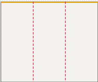
Ściana lewa od lewej: FR-009 ... FR-007, LED 300 × 250 cm plik 303 × 253 cm, spąd 1,5 cm po obrysie, łączeń: 2
