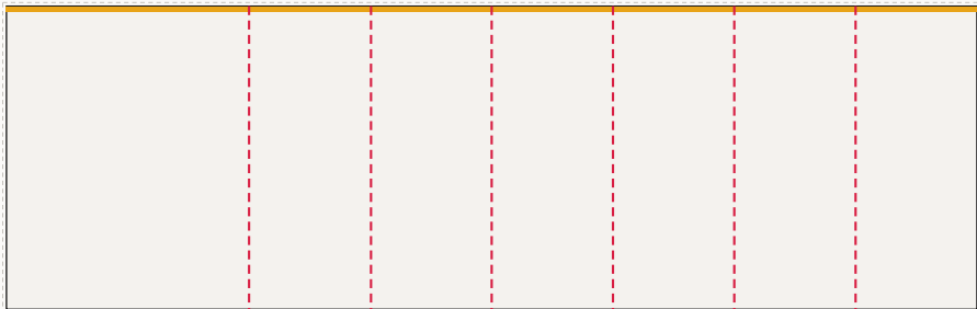
Ściana tylna od lewej: FR-001 ... FR-007, LED 800 × 250 cm plik 803 × 253 cm, spad 1,5 cm po obrysie, łączni: 6
