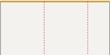
Ściana lewa od lewej: FR-009, FR-007, LED 500 × 250 cm plik 503 × 253 cm, spad 1,5 cm po obrysie, łącząc: 2
