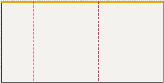
Ściana lewa od lewej: FR-007 ... FR-005, LED 500 × 250 cm plik 503 × 253 cm, spad 1,5 cm po obrysie, łączy: 2
