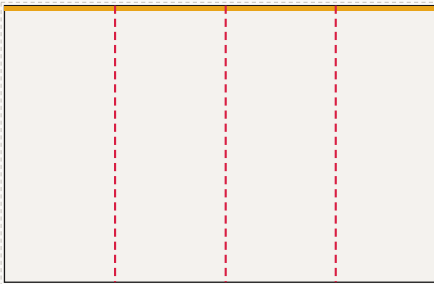
Ściana lewa od lewej: FR-006 ... FR-003, LED 390 × 250 cm plik 393 × 253 cm, spad 1,5 cm po obrysie, łączeń: 3
