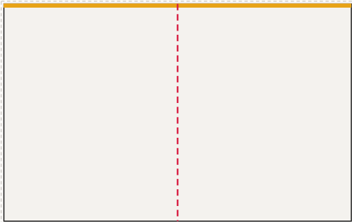
Ściana tylna od lewej: FR-002, FR-003, LED 400 × 250 cm plik 403 × 253 cm, spąd 1,5 cm po obrysie, łączeń: 1
