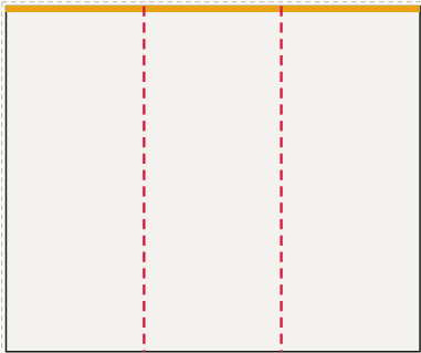
Ściana lewa od lewej: FR-007 ... FR-005, LED 300 × 250 cm plik 303 × 253 cm, spąd 1,5 cm po obrysie, łączeń: 2
