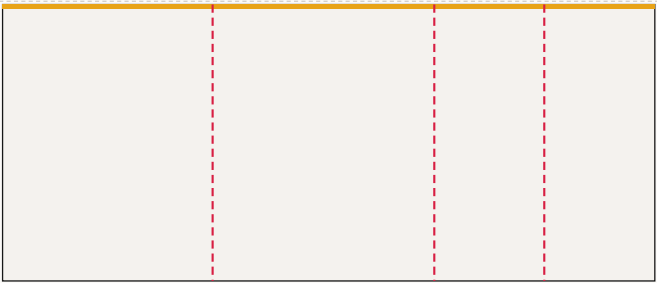
Ściana tylna od lewej: FR-001 ... FR-004, LED 590 × 250 cm plik 593 × 253 cm, spąd 1,5 cm po obrysie, łączeń: 3
