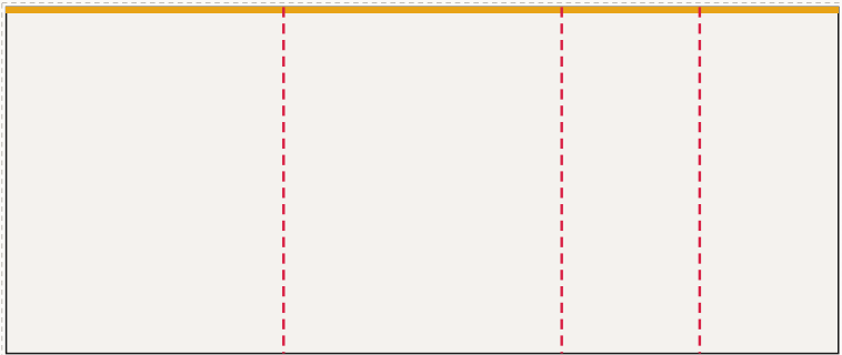
Ściana tylna od lewej: FR-001 ... FR-004, LED 600 × 250 cm plik 603 × 253 cm, spad 1,5 cm po obrysie, łączeń: 3
