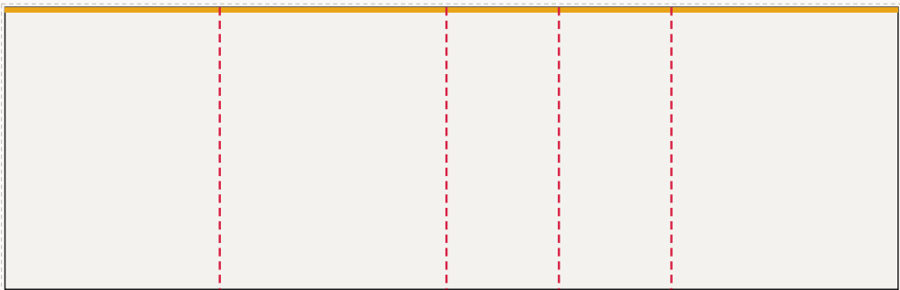
Ściana tylna od lewej: FR-001 ... FR-005, LED 790 × 250 cm plik 793 × 253 cm, spad 1,5 cm po obrysie, łączeń: 4
