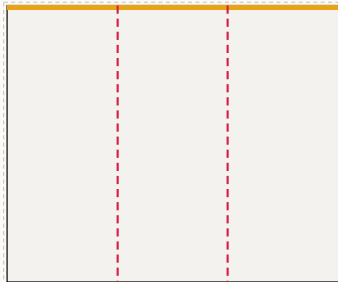
Ściana lewa od lewej: FR-008 ... FR-006, LED 300 × 250 cm plik 303 × 253 cm, spad 1,5 cm po obrysie, łączeń: 2
