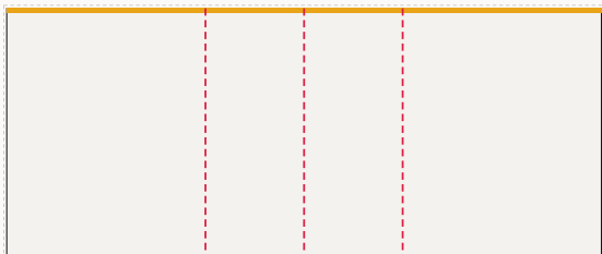
Ściana tylna od lewej: FR-002 ..., FR-005, LED 600 × 250 cm plik 603 × 253 cm, spad 1,5 cm po obrysie, łączęń: 3
