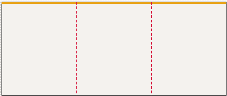
Ściana tylna od lewej: FR-002 ... FR-004, LED 601 × 250 cm plik 604 × 253 cm, spad 1,5 cm po obrysie, łączęń: 2
