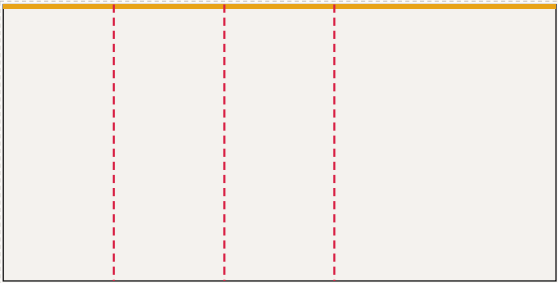
Ściana lewa od lewej: FR-009 ... FR-006, LED 500 × 250 cm plik 503 × 253 cm, spąd 1,5 cm po obrysie, łączeń: 3
