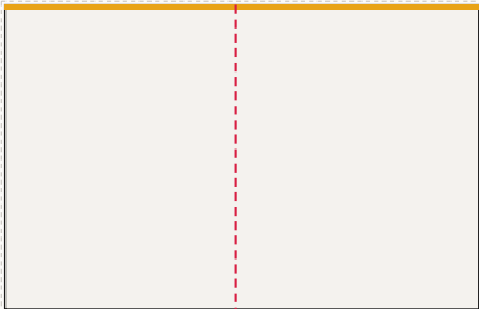
Ściana tylna, część 1 z 2 od lewej: FR-001, FR-002, LED 390 × 250 cm plik 393 × 253 cm, spąd 1,5 cm po obrysie, łączeń: 1
