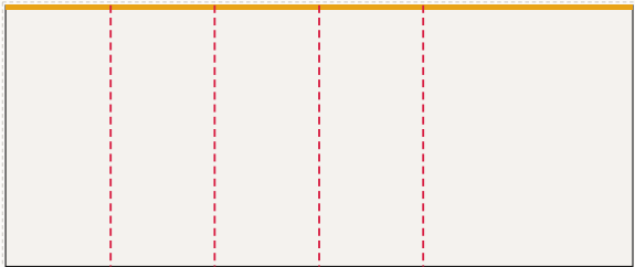
Ściana tylna od lewej: FR-002 ..., FR-006, LED 600 × 250 cm plik 603 × 253 cm, spad 1,5 cm po obrysie, łączęć: 4
