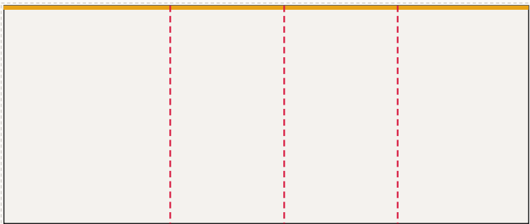
Ściana tylna od lewej: FR-002 ... FR-005, LED 601 × 250 cm plik 604 × 253 cm, spad 1,5 cm po obrysie, łączeń: 3
