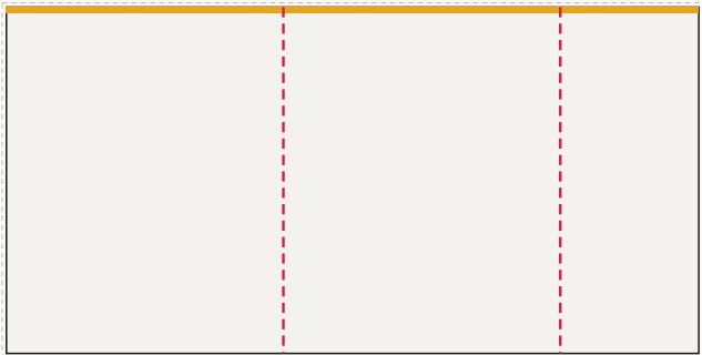
Ściana lewa od lewej: FR-006 ... FR-004, LED 500 × 250 cm plik 503 × 253 cm, spad 1,5 cm po obrysie, łączeń: 2
