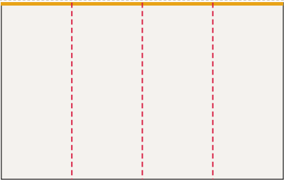
Ściana lewa od lewej: FR-008 ... FR-005, LED 400 × 250 cm plik 403 × 253 cm, spad 1,5 cm po obrysie, łączęć: 3
