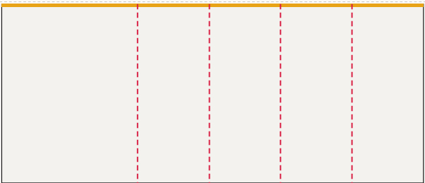
Ściana prawa od lewej: FR-005 ... FR-009, LED 590 × 250 cm plik 593 × 253 cm, spad 1,5 cm po obrysie, łączęń: 4
