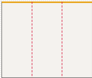
Ściana tylna, część 1 z 2 od lewej: FR-001 ... FR-003, LED 300 × 250 cm plik 303 × 253 cm, spad 1,5 cm po obrysie, łączni: 2
