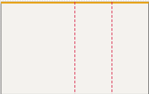
Ściana prawa od lewej: FR-009 ... FR-011, LED 400 × 250 cm plik 403 × 253 cm, spad 1,5 cm po obrysie, łączęć: 2
