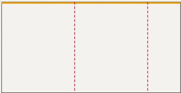
Ściana tylna od lewej: FR-001 ... FR-003, LED 490 × 250 cm plik 493 × 253 cm, spad 1,5 cm po obrysie, łączeń: 2
