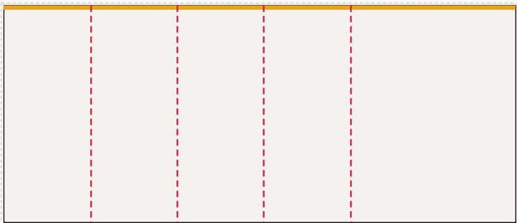
Ściana tylna od lewej: FR-001 ... FR-005, LED 590 × 250 cm plik 593 × 253 cm, spad 1,5 cm po obrysie, łączeń: 4
