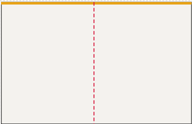
Ściana prawa od lewej: FR-005, FR-006, LED 390 × 250 cm plik 393 × 253 cm, spad 1,5 cm po obrysie, łączący: 1
