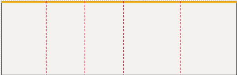
Ściana tylna od lewej: FR-001 ... FR-005, LED 791 × 250 cm plik 794 × 253 cm, spad 1,5 cm po obrysie, łączeń: 4
