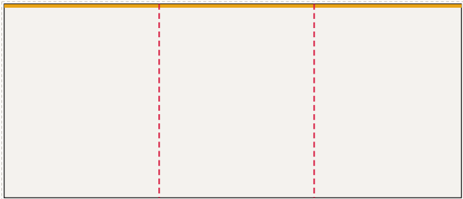
Ściana tylna od lewej: FR-001 ... FR-003, LED 590 × 250 cm plik 593 × 253 cm, spad 1,5 cm po obrysie, łączeń: 2
