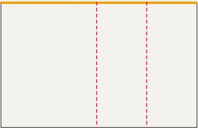
Ściana prawa od lewej: FR-004 ... FR-006, LED 390 × 250 cm plik 393 × 253 cm, spad 1,5 cm po obrysie, łączeń: 2
