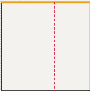
Ściana prawa od lewej: FR-004, FR-005, LED 250 × 250 cm plik 253 × 253 cm, spad 1,5 cm po obrysie, łączeń: 1
