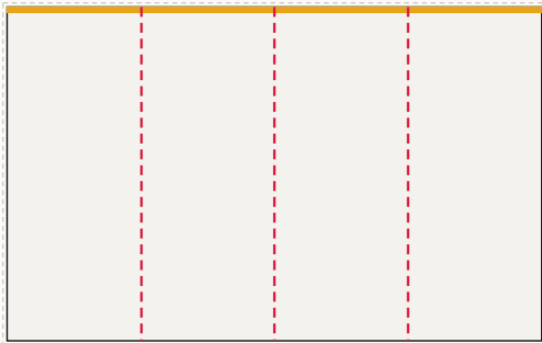
Ściana prawa od lewej: FR-006 ... FR-009, LED 400 × 250 cm plik 403 × 253 cm, spad 1,5 cm po obrysie, łączeń: 3
