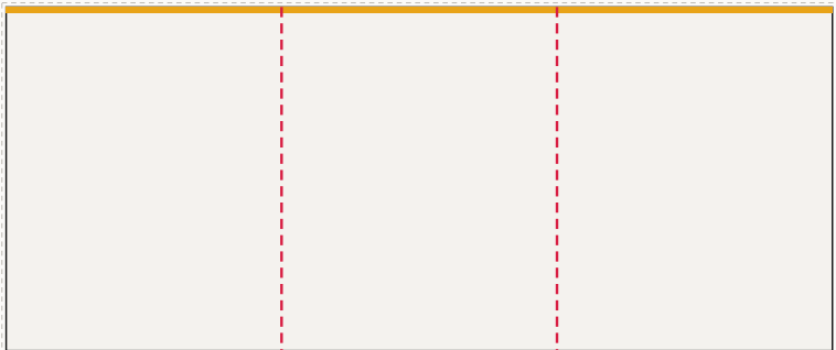
Ściana tylna od lewej: FR-001 ... FR-003, LED 600 × 250 cm plik 603 × 253 cm, spad 1,5 cm po obrysie, łączień: 2
