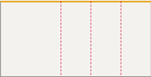
Ściana prawa od lewej: FR-005 ..., FR-008, LED 500 × 250 cm plik 503 × 253 cm, spad 1,5 cm po obrysie, łączeń: 3
