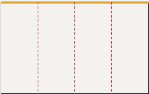
Ściana tylna, część 2 z 2 od lewej: FR-005 ... FR-008, LED 400 × 250 cm plik 403 × 253 cm, spad 1,5 cm po obrysie, łączeń: 3
