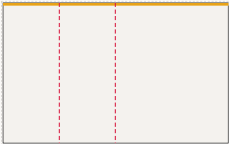
Ściana tylna, część 1 z 2 od lewej: FR-001 ... FR-003, LED 400 × 250 cm plik 403 × 253 cm, spad 1,5 cm po obrysie, łączęń: 2
