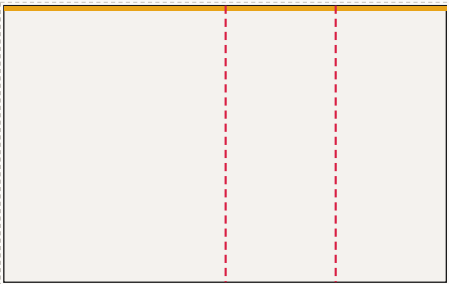
Ściana tylna, część 2 z 2 od lewej: FR-004 ... FR-006, LED 400 × 250 cm plik 403 × 253 cm, spad 1,5 cm po obrysie, łączęń: 2
