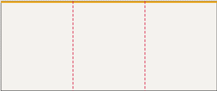
Ściana tylna od lewej: FR-001 ... FR-003, LED 600 × 250 cm plik 603 × 253 cm, spad 1,5 cm po obrysie, łączeń: 2
