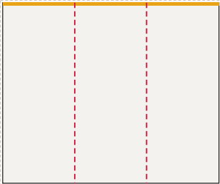
Ściana tylna, część 1 z 2 od lewej: FR-001 ... FR-003, LED 300 × 250 cm plik 303 × 253 cm, spad 1,5 cm po obrysie, łączęci: 2
