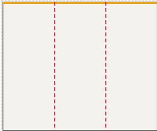
Ściana tylna, część 2 z 2 od lewej: FR-004 ... FR-006, LED 300 × 250 cm plik 303 × 253 cm, spad 1,5 cm po obrysie, łączęci: 2
