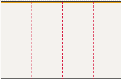
Ściana lewa od lewej: FR-007 ... FR-004, LED 390 × 250 cm plik 393 × 253 cm, spad 1,5 cm po obrysie, łączef: 3
