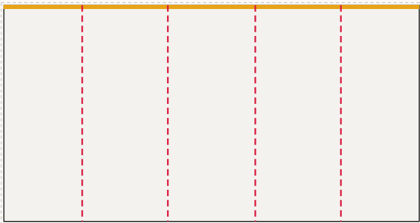
Ściana tylna od lewej: FR-001 ... FR-005, LED 480 × 250 cm plik 483 × 253 cm, spąd 1,5 cm po obrysie, łączni: 4
