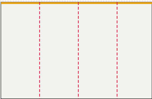
Ściana lewa od lewej: FR-009 ... FR-006, LED 390 × 250 cm plik 393 × 253 cm, spad 1,5 cm po obrysie, łączni: 3
