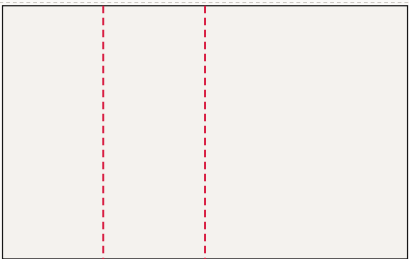
Ściana lewa od lewej: FR-011 ... FR-009 400 × 250 cm plik 403 × 253 cm, spad 1,5 cm po obrysie, łączęń: 2
