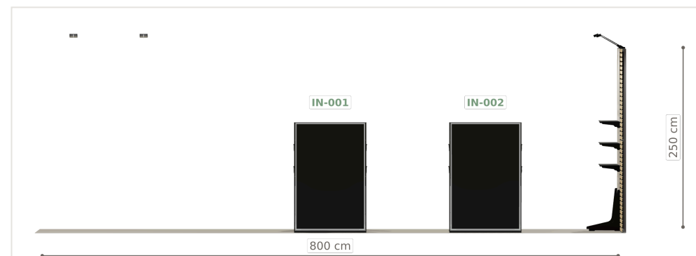
ELEWACJA 4
