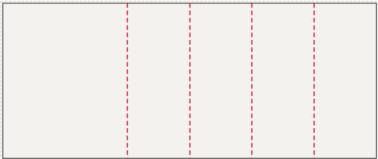
Ściana tylna od lewej: FR-001 ... FR-005 600 × 250 cm plik 603 × 253 cm, spad 1,5 cm po obrysie, łączeń: 4
